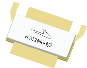
PXFE181507FC Package H-37248G-4/2
